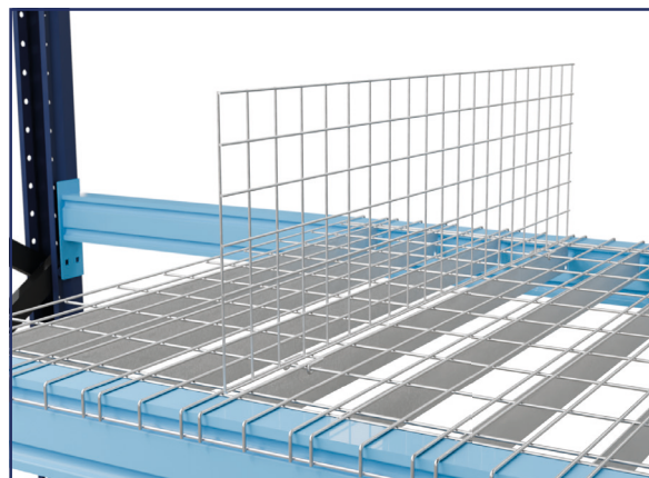
GIDRA® PART DGB Einbausituation
